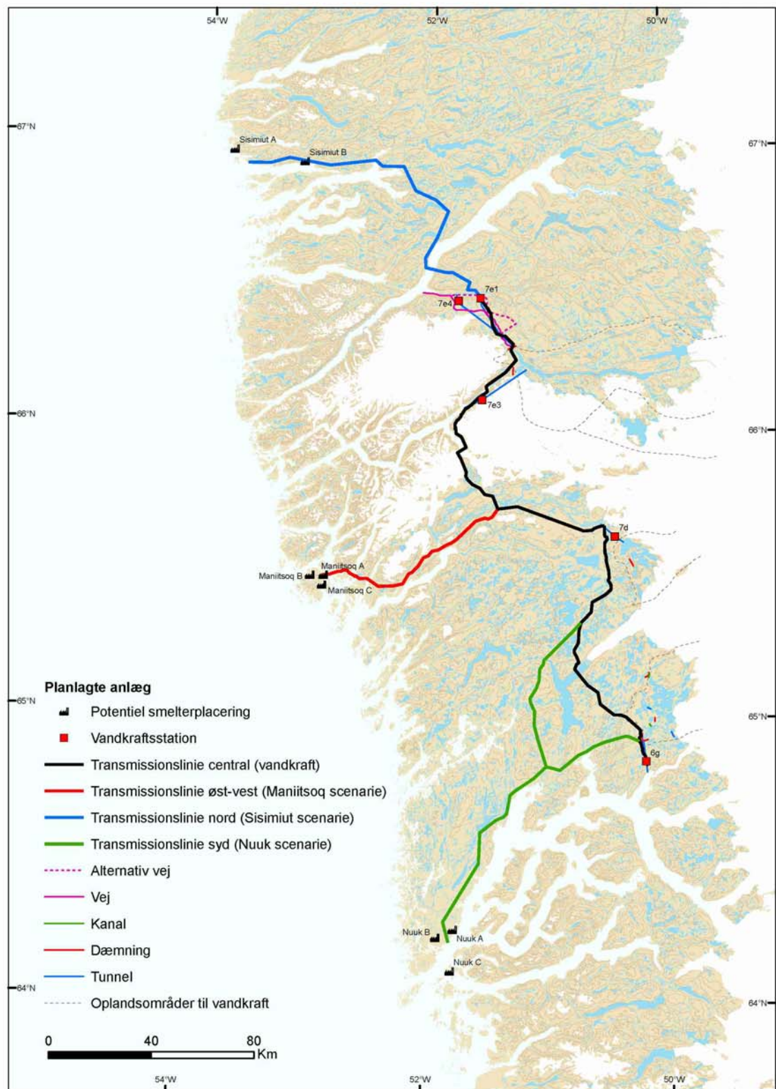
Figur 1.1. Anlæg i forbindelse med vandkraft og aluminiumssmelter.
