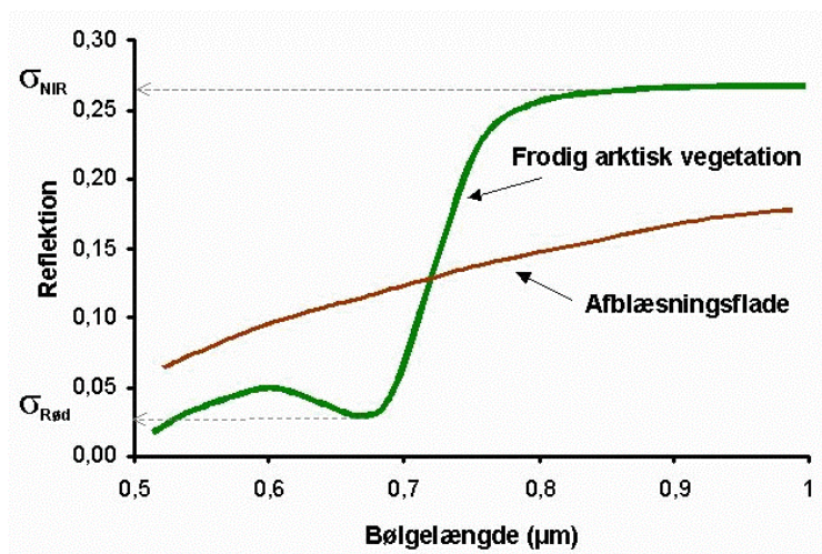
Figur 2.5. Spektralsignatur for en frodig arktisk vegetation (kær domineret af polar-kæruld) vist ved den grønne kurve og for en arktisk afblæsningsflade vist ved den brune kurve. Det typiske spring i vegetationskurven ved 0,75µm skyldes klorofyl og cellestruktur, og kaldes for vegetationspringet. Pilene angiver refleksionen af sollys fra den frodige arktiske vegetation for henholdsvis den nærinfrarøde ( \sigma_{\text{NIR}} ) og det røde ( \sigma_{\text{Rød}} ) spektre.
